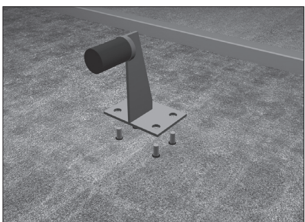
На анкерные болты наденьте основание корпуса бокового упора.
