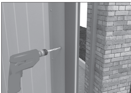
Просверлите 2 отверстия \varnothing 12 в створке.
